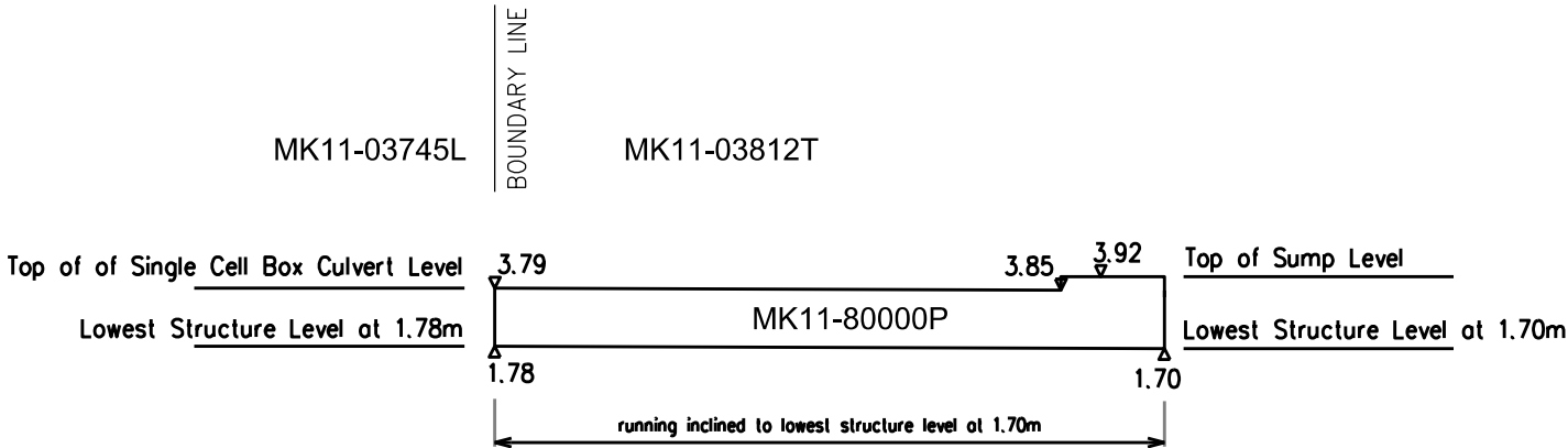
SECTION E1-E1
