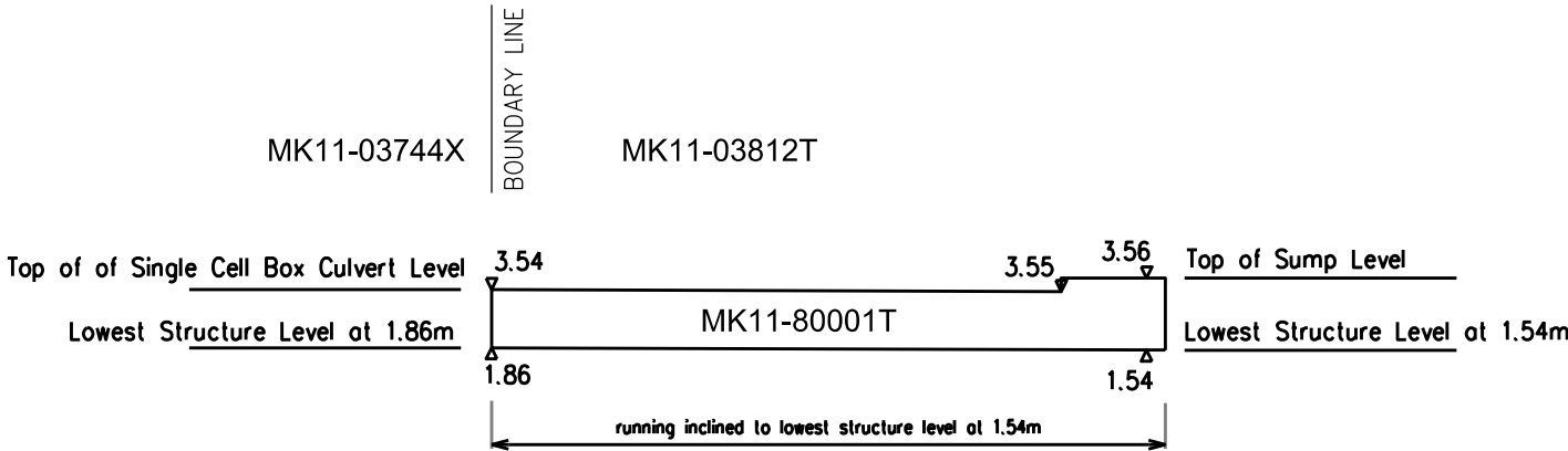
SECTION E2-E2
